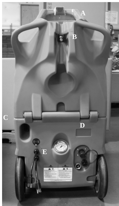
FIG. 2 : Vue arrière
